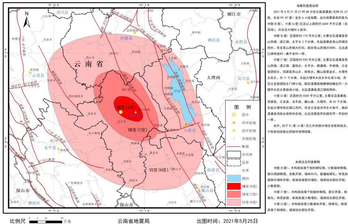
云南漾濞6.4级地震烈度图
